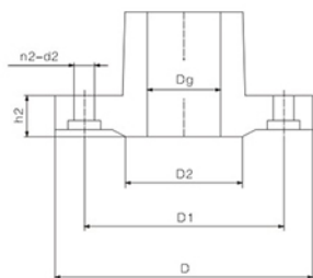
连接法兰
